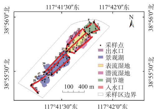
图1 天津临港湿地采样点布设
