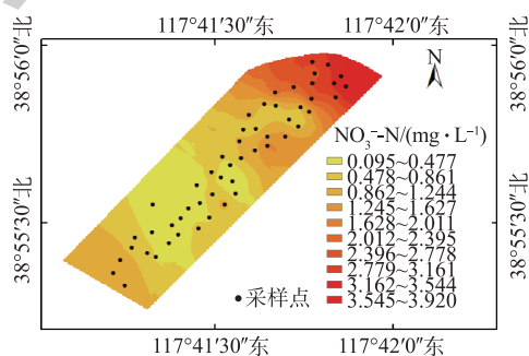
图5 湿地 \text{NO}_3^-\text{-N} 的分布
